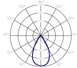
■ C0-C180 ■ C90-C270 ed/1000lm
