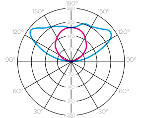
■ C0-C180 ■ C90-C270 ed/1000lm
